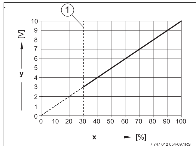
Рис. 14 Клемма U_{BR}
